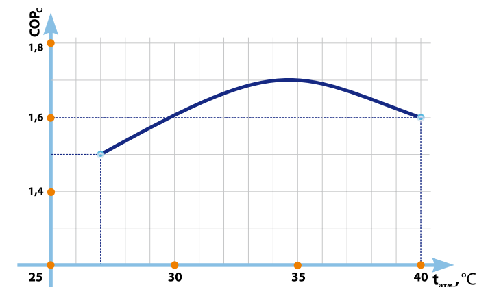
Рис. 2. Эффективность ВКС в режиме кондиционирования при 100% подаче свежего воздуха.
