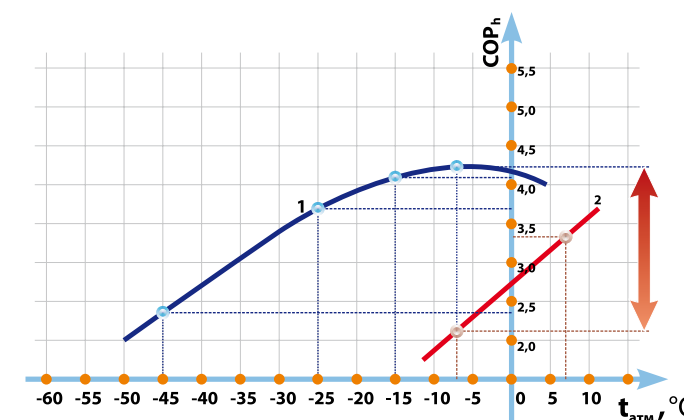
Рис. 1. Сравнение ВКС (1) и фреонового теплового насоса (2) в режиме отопления.
